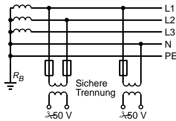
Abb. 24: SELV
