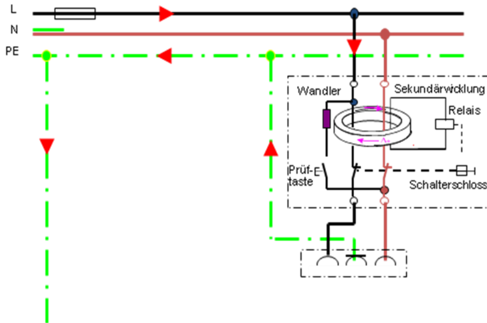
Abb. 27: Funktion einer Fehlerstrom-Schutzeinrichtung (RCD)
