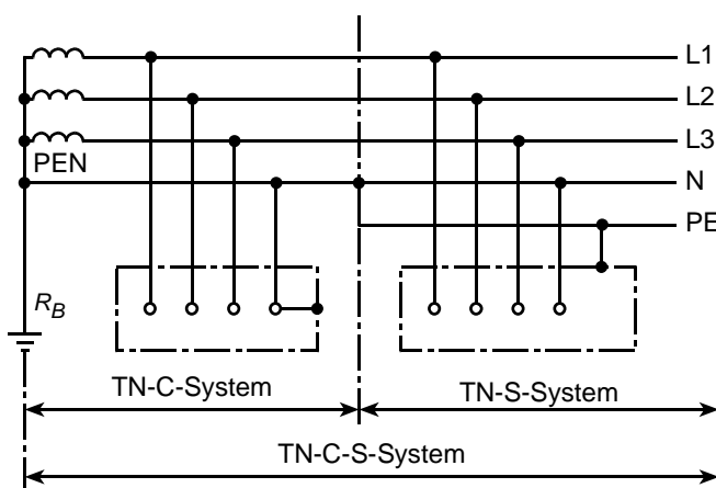
Abb. 15: a) TN-C-S-System
