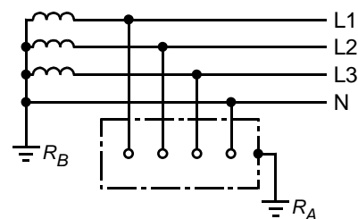
Abb. 16: b) TT-System
