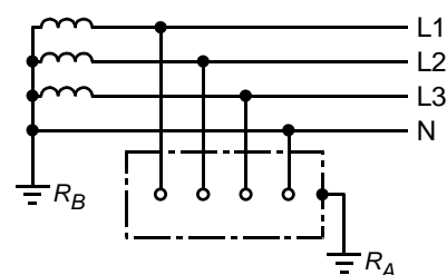
Abb. 16: b) TT-System
